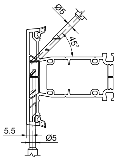
770365 імпост 82 мм
