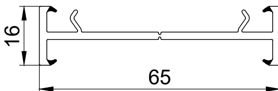
552300 з'єднувач Н-подібний
