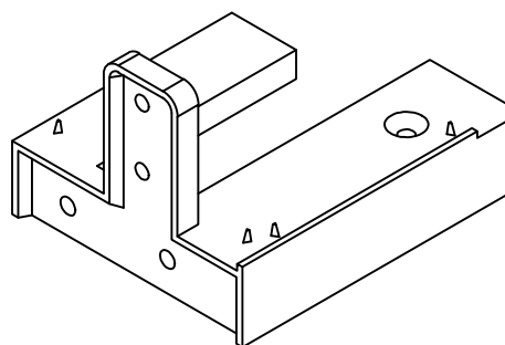
77-26 з'єднувач порога ширина 76 мм (пара)
