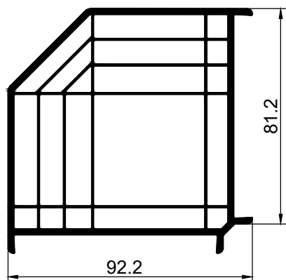
771665 з'єднувач 90°
