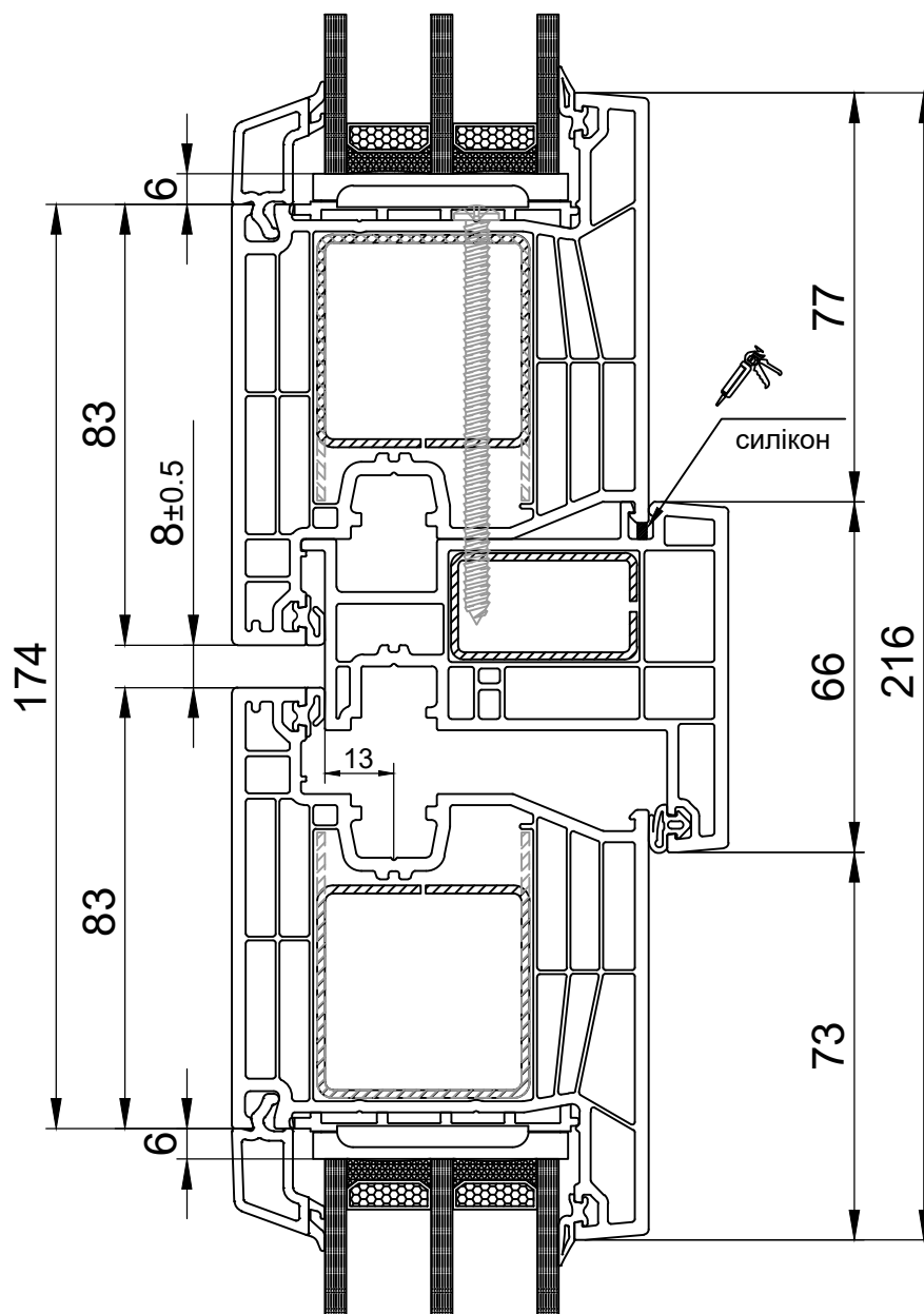
СХЕМА 771265 ШТУЛЬП 770565 ДВЕРНА СТУЛКА 104 мм
