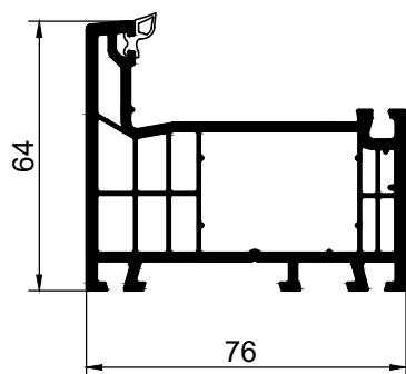
770165 рама 64 мм
