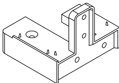
77-25 з'єднувач порога ширина 76 мм (пара)
