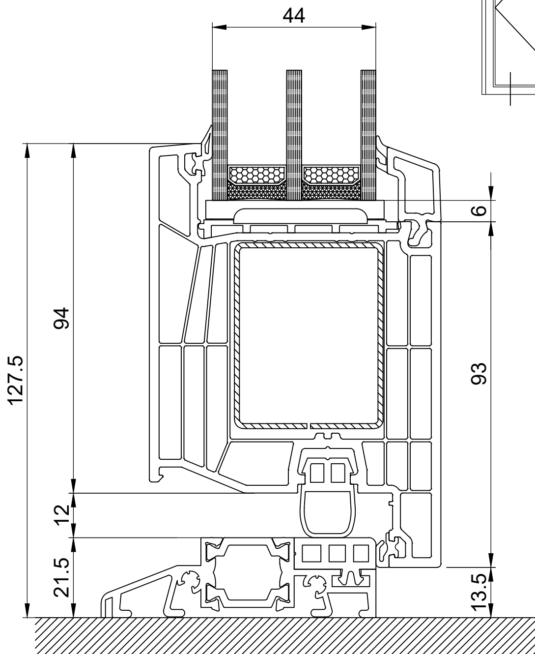
СХЕМА 772565 СТУЛКА ДВЕРНА 114 мм ПОРІГ АЛЮМІНІЄВИЙ З ТЕРМОМОСТОМ
