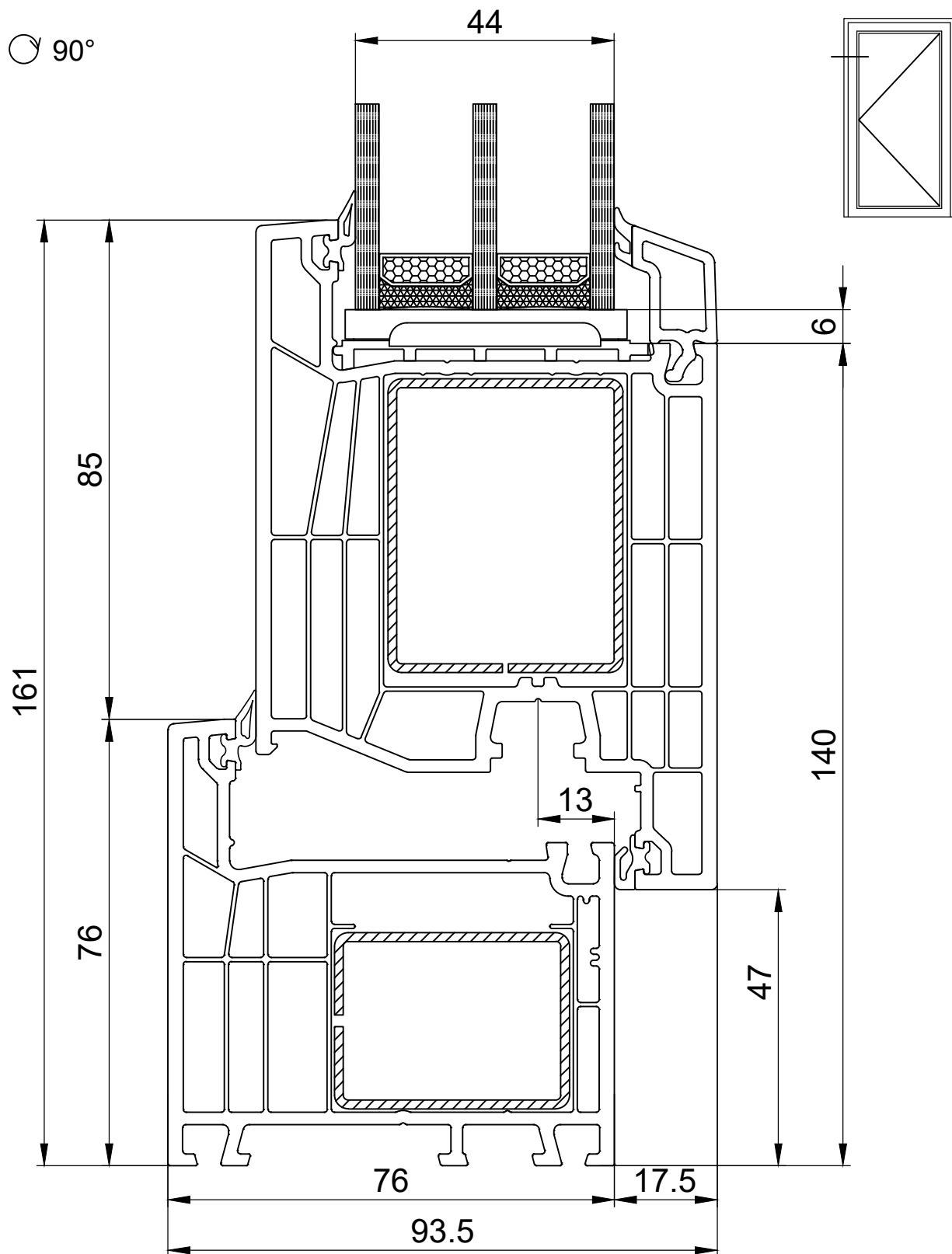
СХЕМА 770665 РАМА 76 мм 772565 СТУЛКА ДВЕРНА 114 мм
