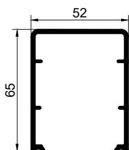
552265 кришка зовнішнього статичного підсилювача
