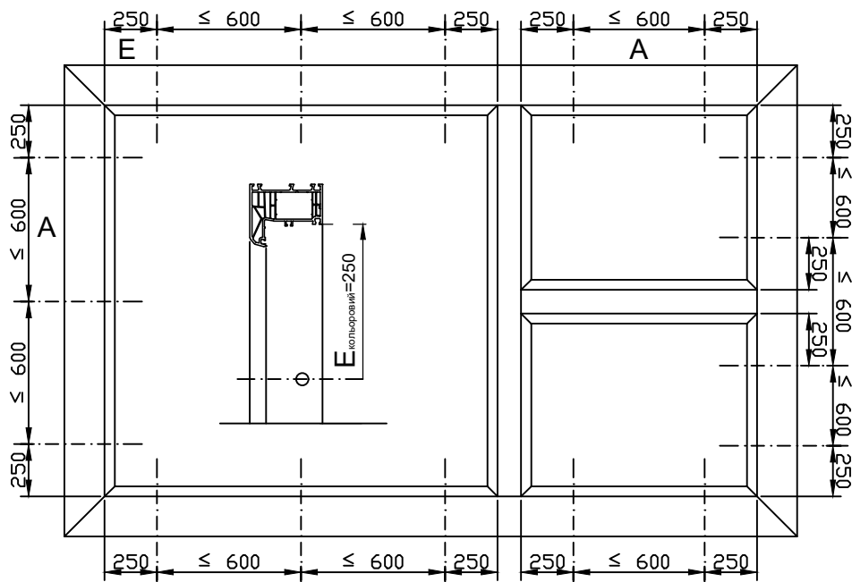
відстань між елементами кріплення для кольорових профілів
