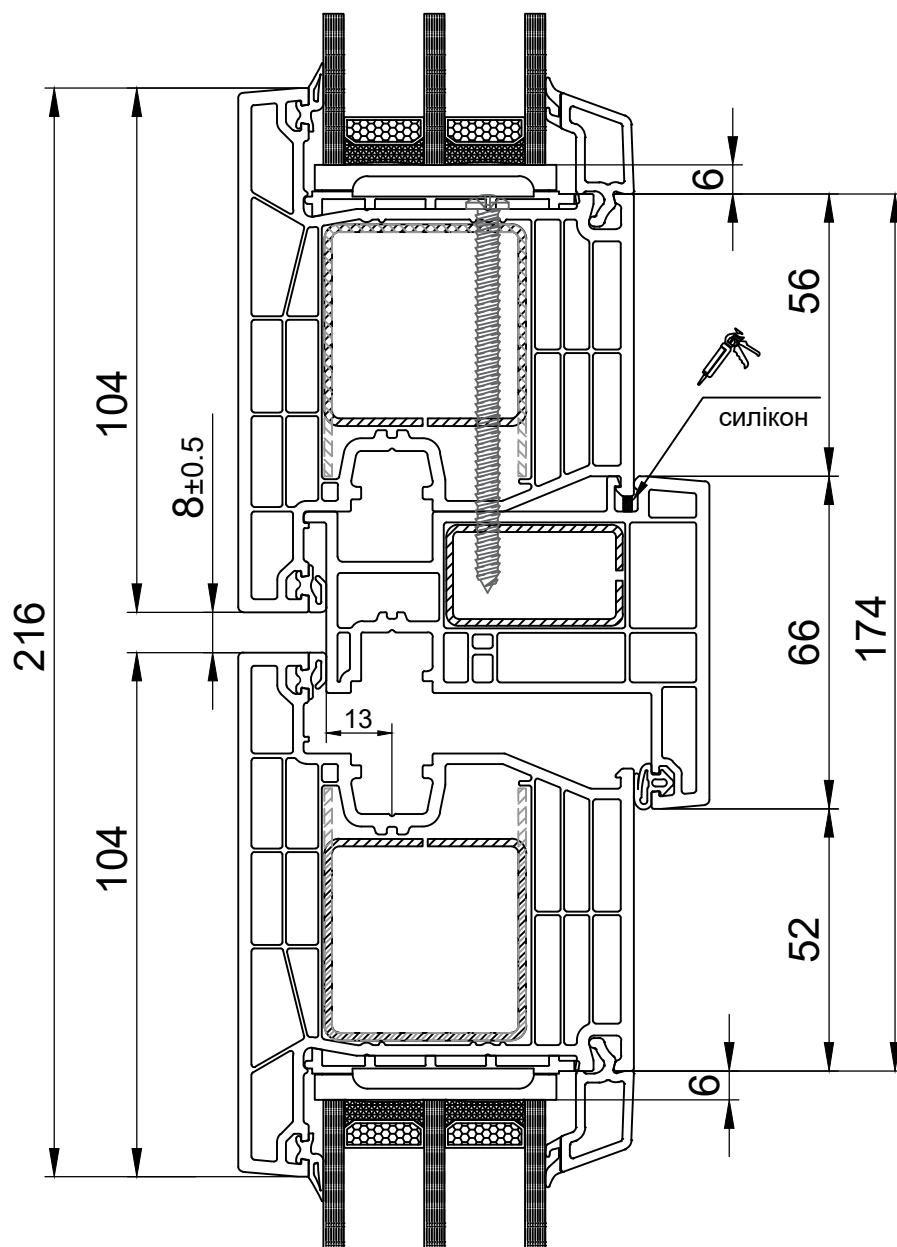
СХЕМА 771265 ШТУЛЬП 770465 ДВЕРНА Т-СТУЛКА 104 мм
