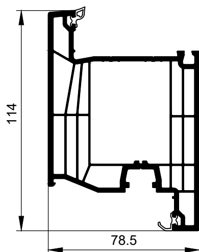
772565 стулка дверна 114 мм
