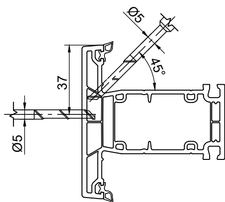
770365 імпост 82 мм
