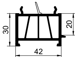
551165 VL профіль підставочний
