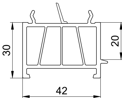
551165 VL профіль підставковий
