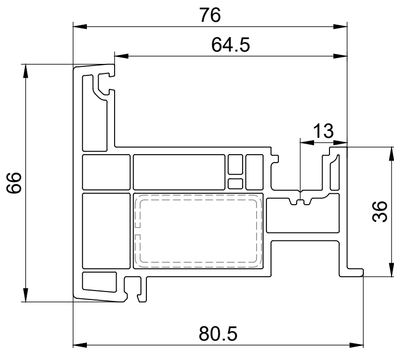
771265 штульп
