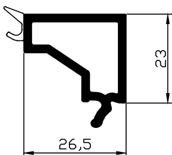
773265 штапик під заповнення 32 мм
