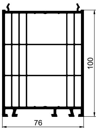
771965 розширювач 100 мм
