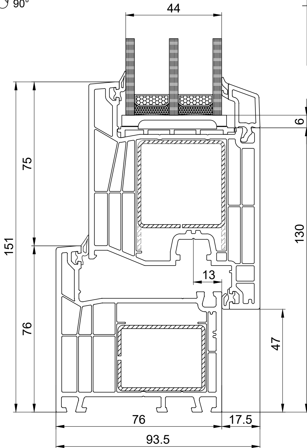
СХЕМА 770665 РАМА 76 мм 770565 СТУЛКА ДВЕРНА 104 мм
