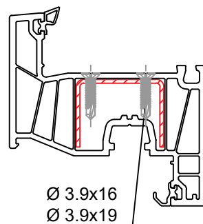
770265 стулка віконна 77 мм
