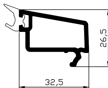
201165 штапик під заповнення 24 мм
