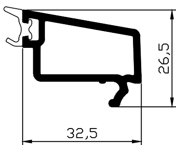
201065 штапик під заповнення 26 мм
