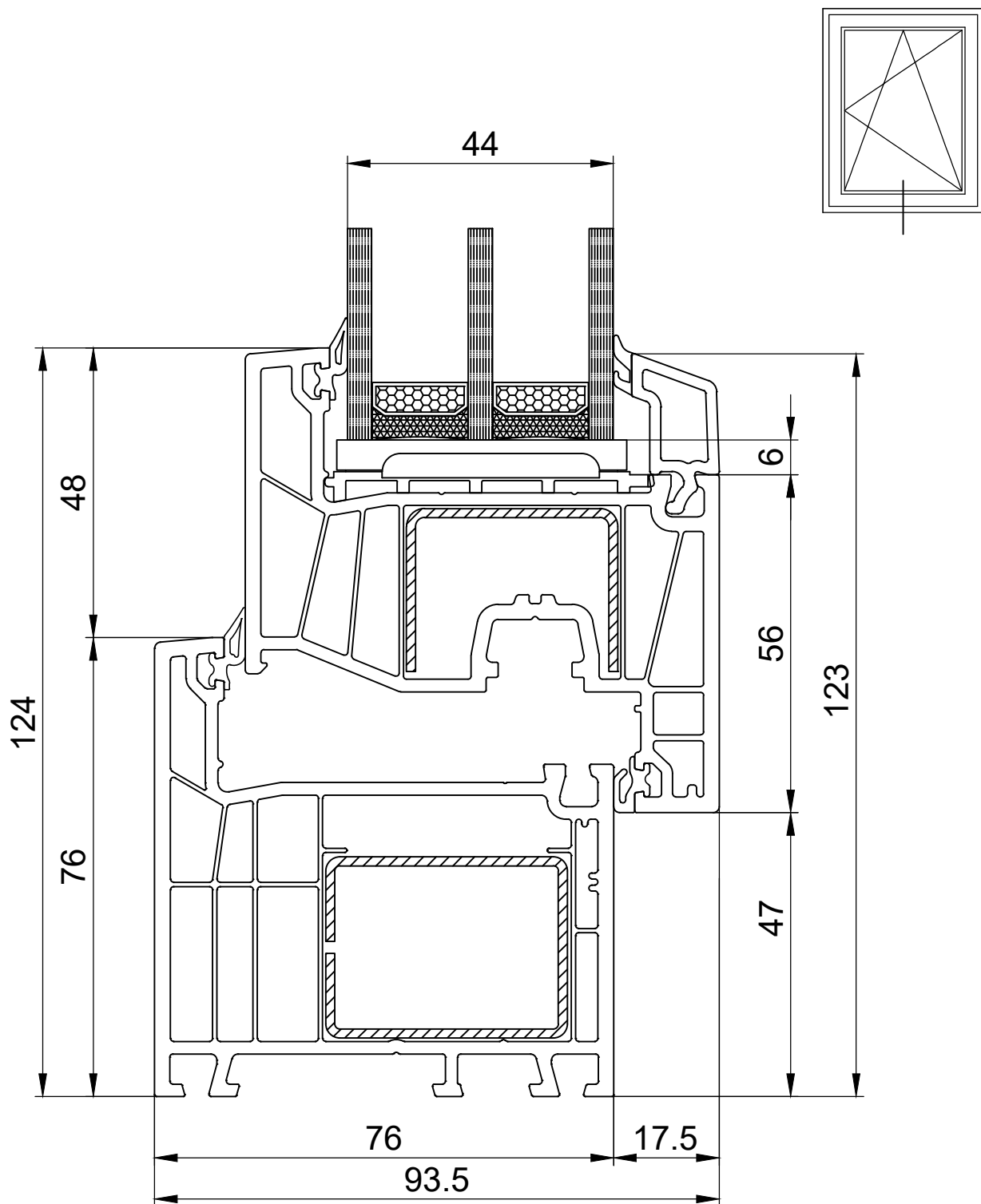
СХЕМА 770665 РАМА 76 мм 770265 СТУЛКА 77 мм
