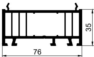
771765 розширювач 35 мм
