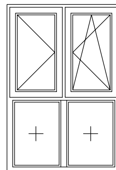
двостулкове поворотно/ відкривання з глухим склінням нижньої частини
