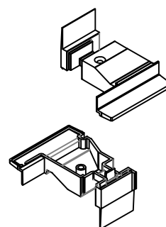
77-07 заглушки штульпа (пара)
