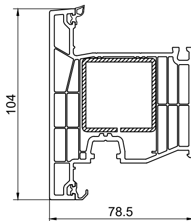
770465 стулка дверна 104 мм
