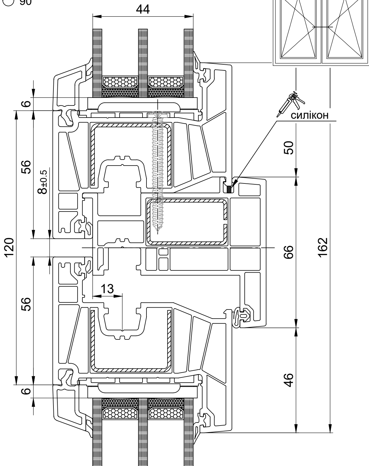
СХЕМА 771265 ШТУЛЬП 770265 СТУЛКА 77 мм
