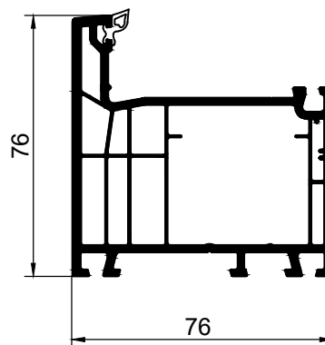
770665 рама 76 мм
