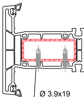
770365 імпост 82 мм
