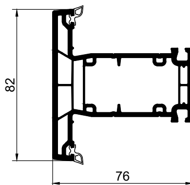
770365 імпост 82 мм
