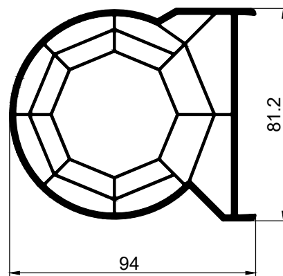
771565 єркер
