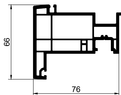
771265 шульп
