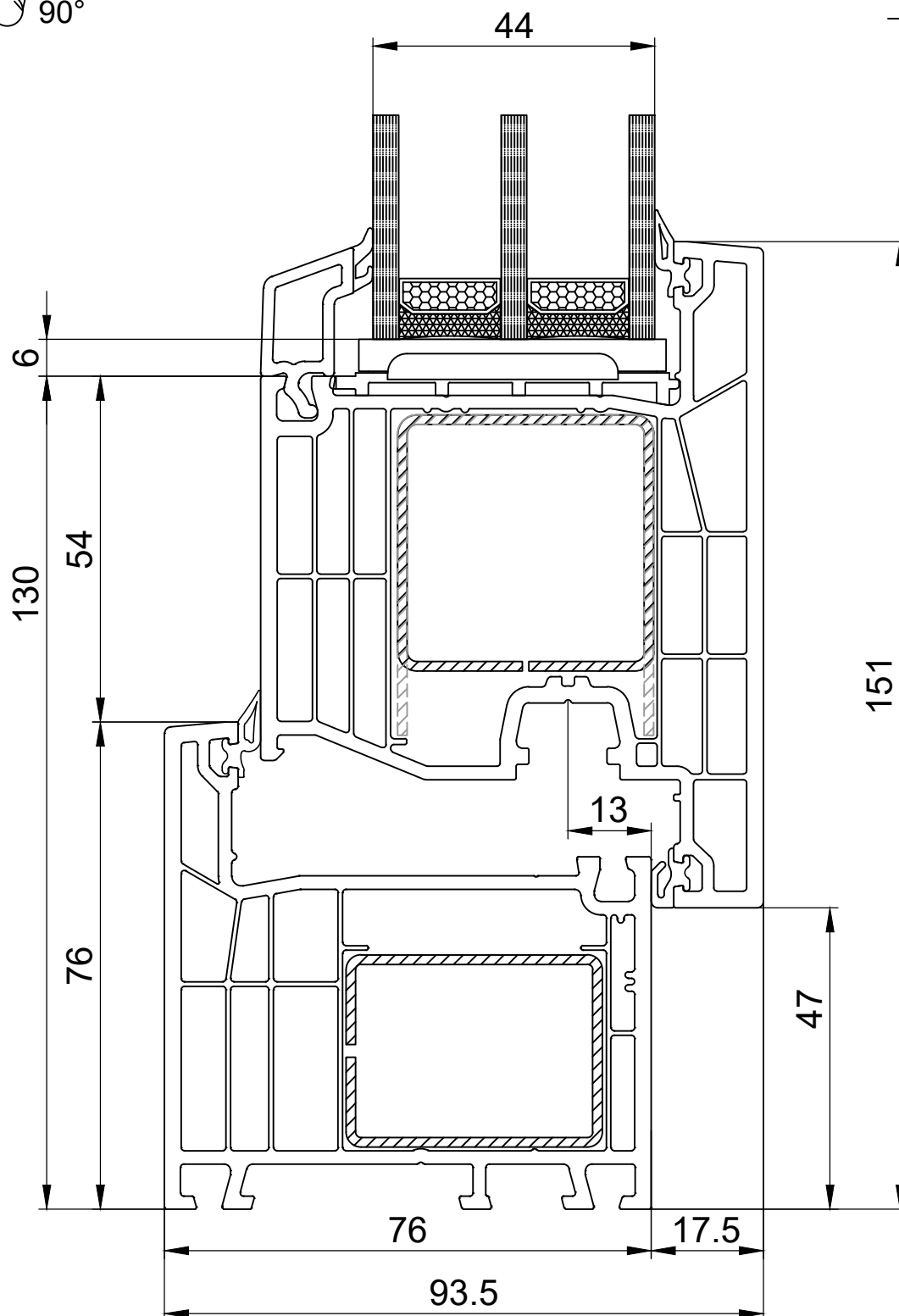
СХЕМА 770665 РАМА 76 мм 770465 Т-СТУЛКА ДВЕРНА 104 мм
