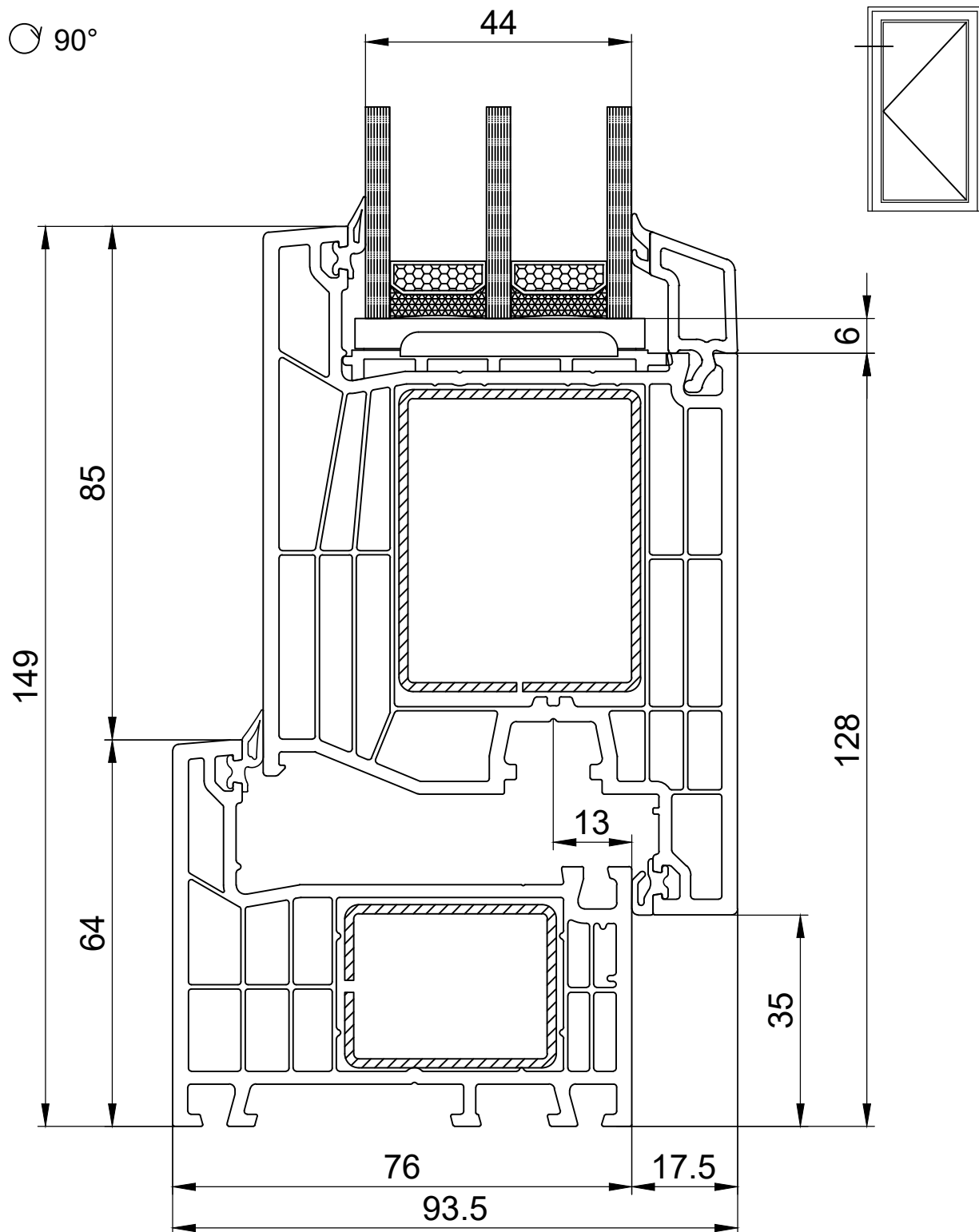
СХЕМА 770165 РАМА 64 мм 772565 СТУЛКА ДВЕРНА 114 мм
