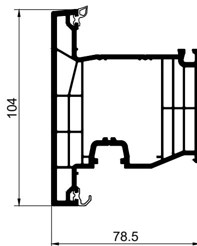
770465 стулка дверна 104 мм
