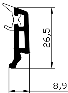
200965 штапик під заповнення 52 мм
