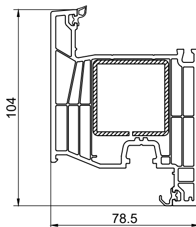
770565 стулка дверна 104 мм
