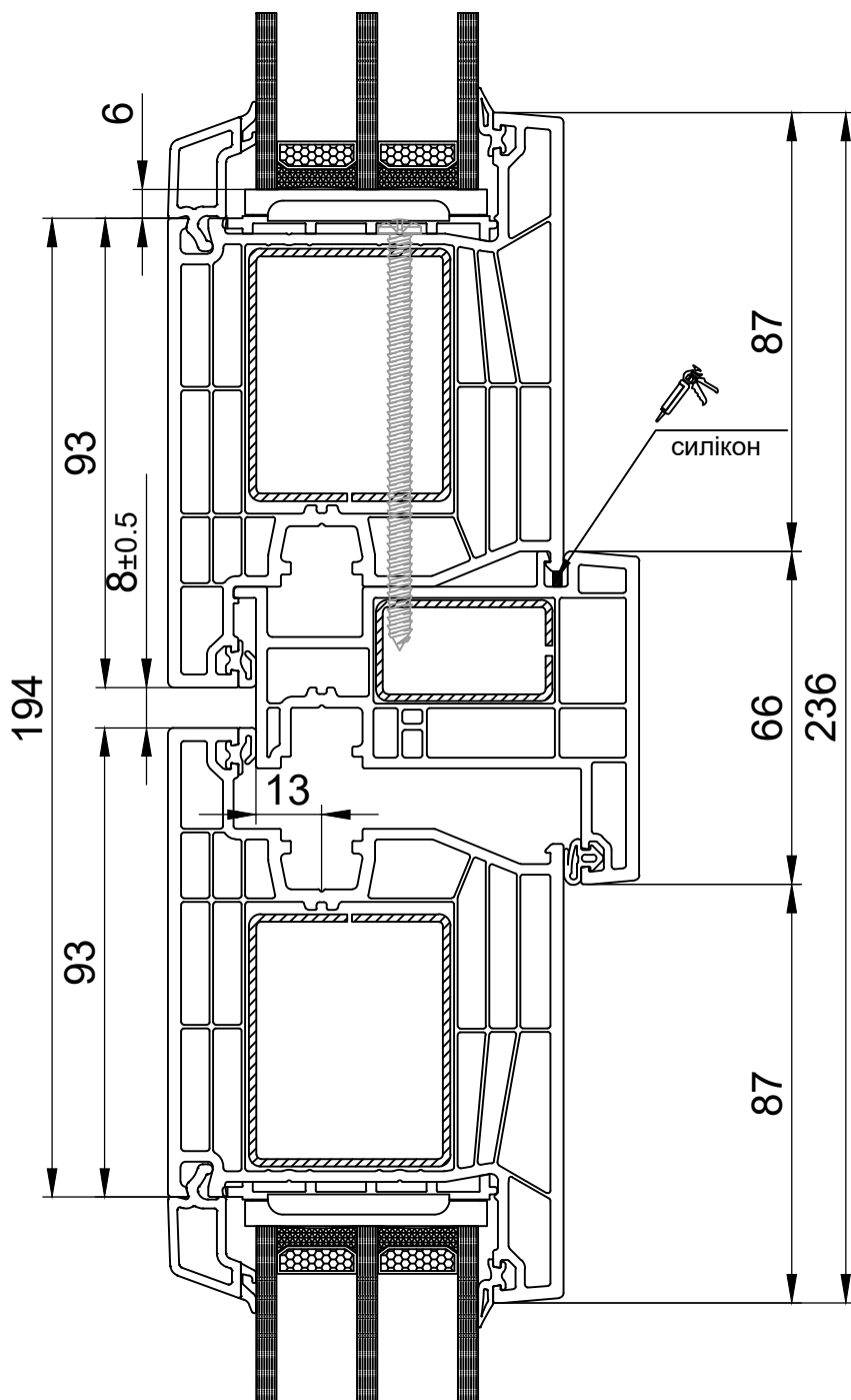
СХЕМА 771265 ШТУЛЬП 772565 ДВЕРНА СТУЛКА 114 мм
