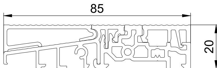
порог TS88510-FL+TSA8851
