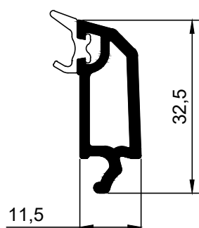
854865 штапик под заполнение 48мм
