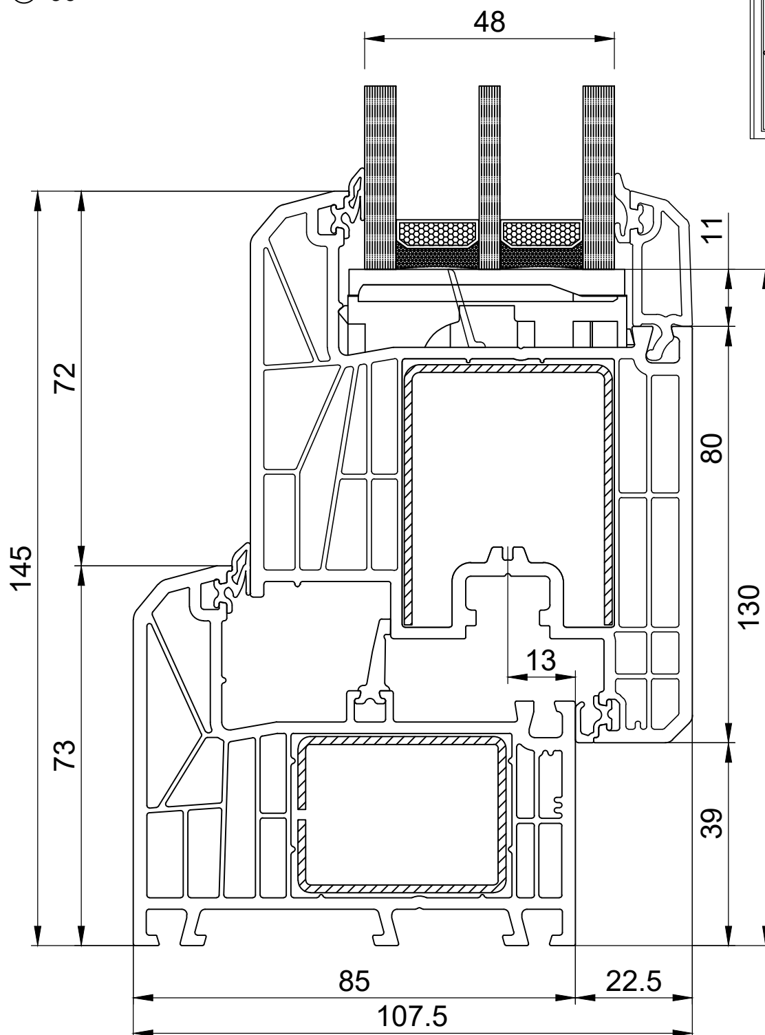
СХЕМА УЗЛА 850165 РАМА 73мм 850565 СТВОРКА ДВЕРНАЯ 106мм
