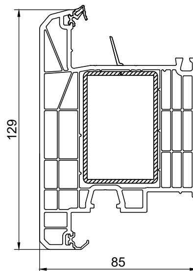
850465 створка дверная 129мм
