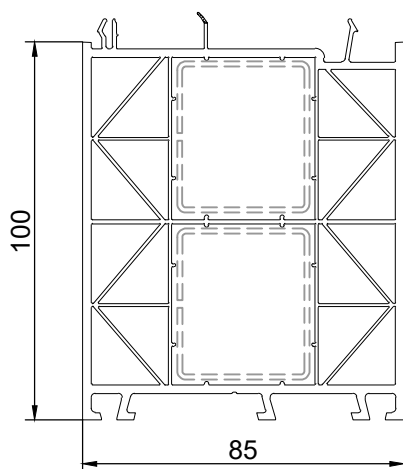
180204 расширитель 100мм
