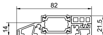
порог алюминиевый анодированный (с термомостом)
