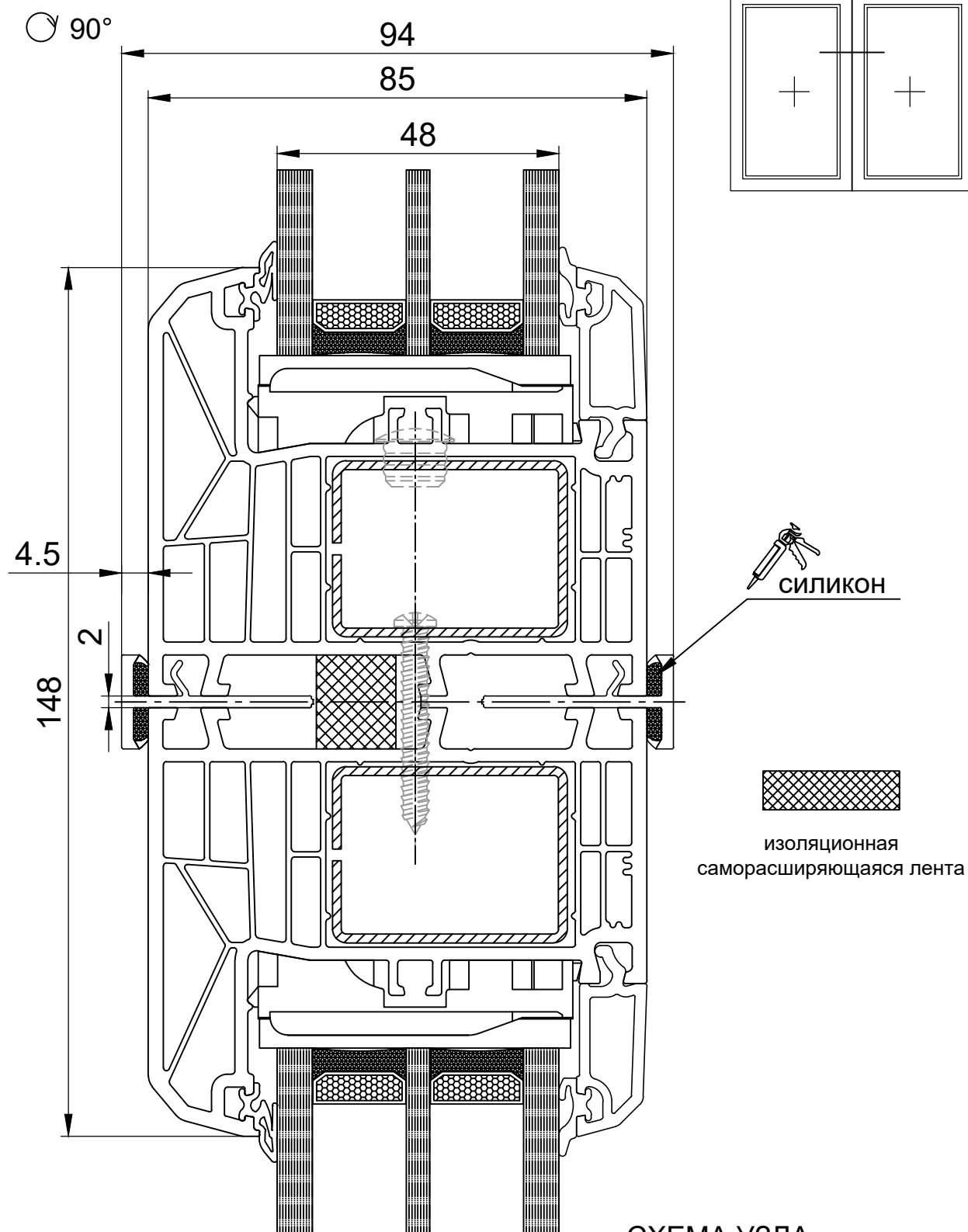
СХЕМА УЗЛА 850165 РАМА 73 мм 552300 соединитель Н-образный 850165 РАМА 73 мм
