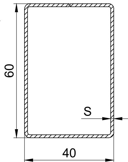
85-04 усилитель углов дверной створки (60x40)
