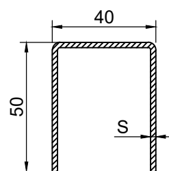
арм. 50x40x50x2.0
