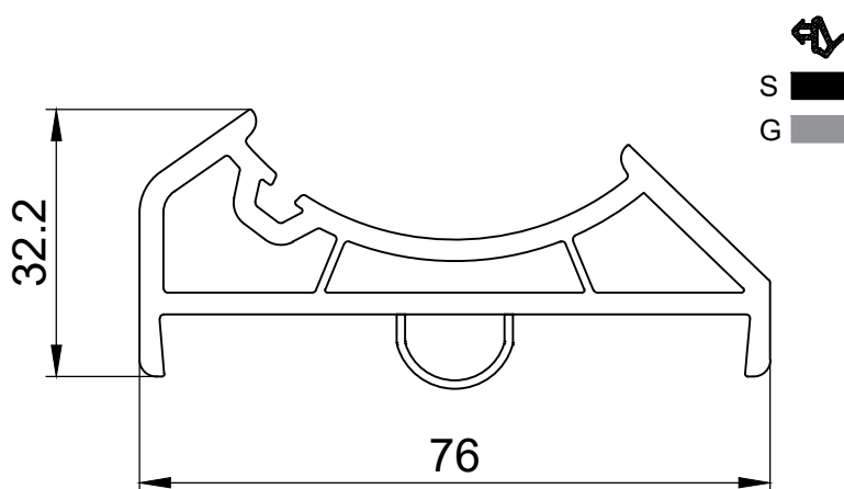
551465 адаптер эркера
