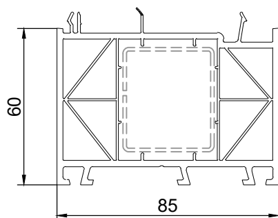
180203 расширитель 60мм
