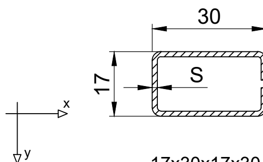
17x30x17x30
