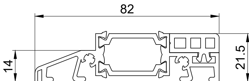
порог алюминиевый анодированный (с термомостом)
