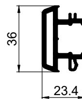
112065 соединитель статический
