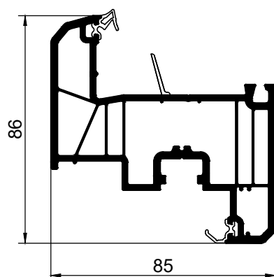
852265 створка оконная 86мм
