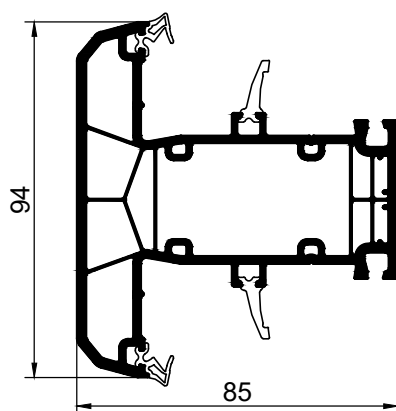
852365 импост 94мм
