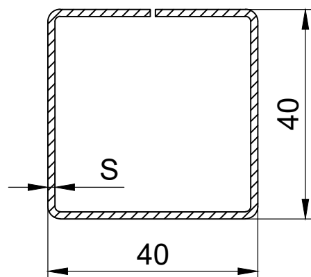
C-обр. 12x40x40x40x12
