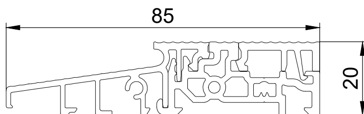
порог TS88510-FL
