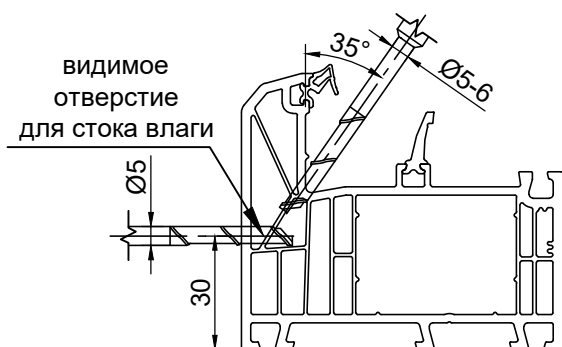
850165 рама 73мм
