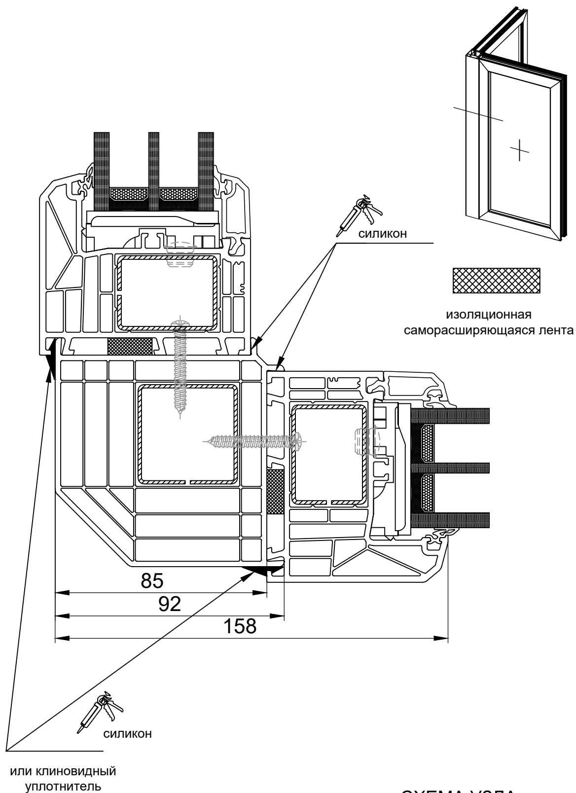
СХЕМА УЗЛА 850165 РАМА 73 мм 771665 соединитель 90° 850165 РАМА 73 мм
