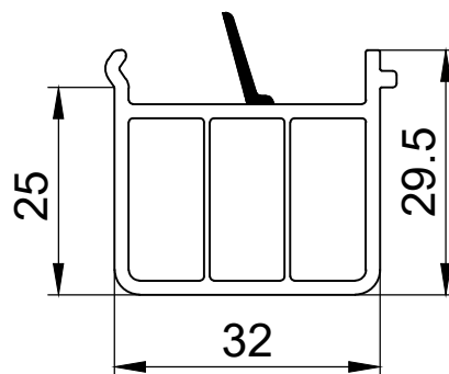
111165 профиль подставочный
