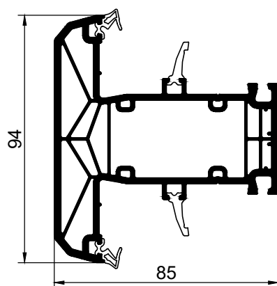
850365 импост 94мм
