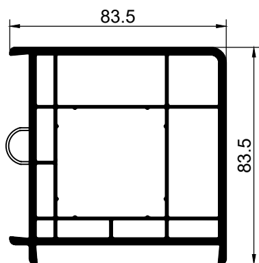
551665 соединитель 90°
