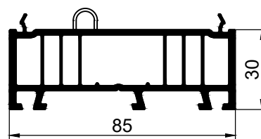
851765 расширитель 30мм
