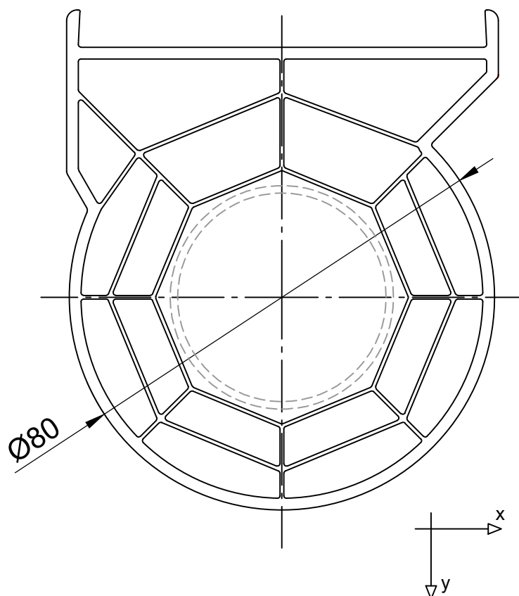
771565 эрек
