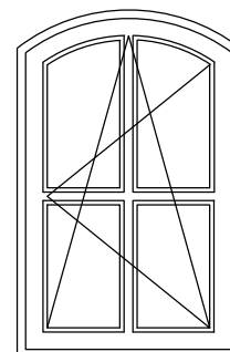
поворотно - откидное открытие конструкции в виде лучковой арки с крестовым импостом в створке
