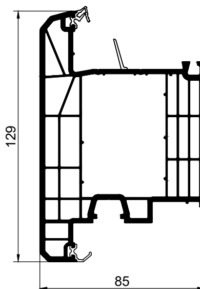
850465 створка дверная 129мм
