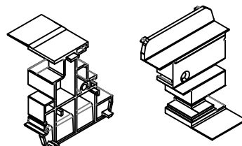
85-07 заглушки штапика (пара)
