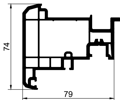
851265 штыль
