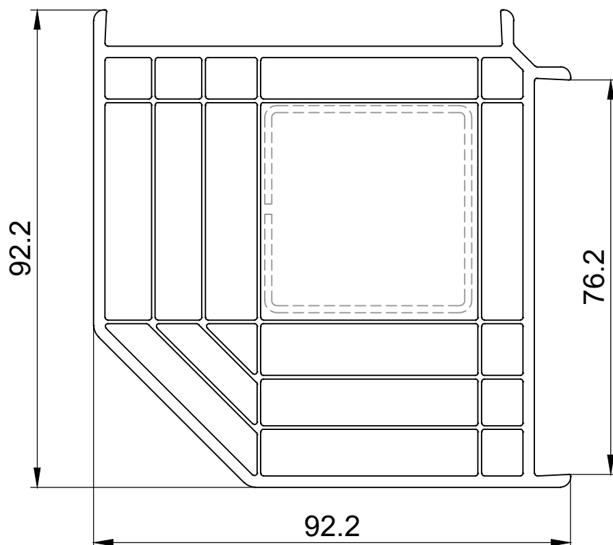
771665 соединитель 90°
