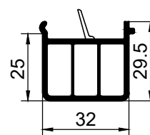
111165 профиль подставочный
