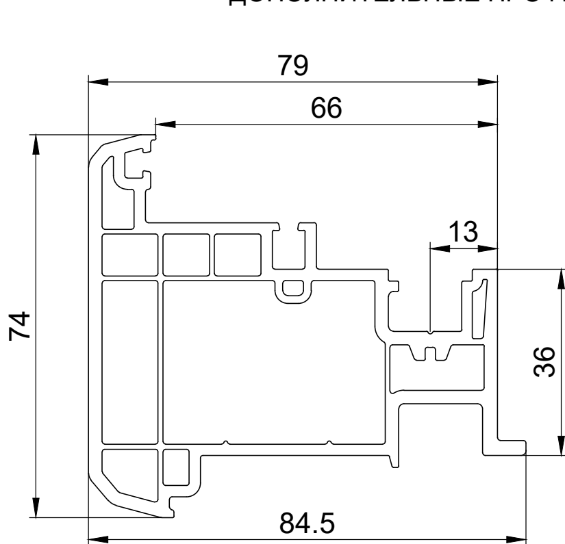
851265 штульп
