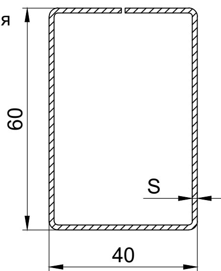
C-обр. 12x60x40x60x12
